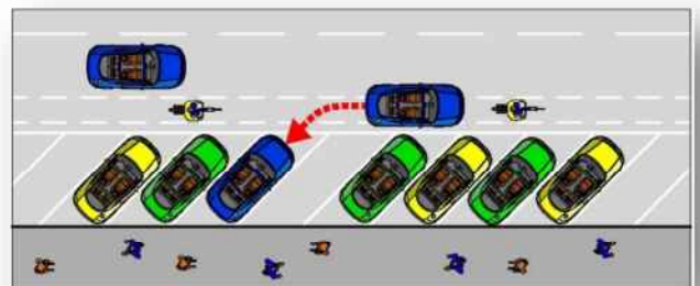
Esempio di funzionamento della sosta a 45° 'retroversa'
